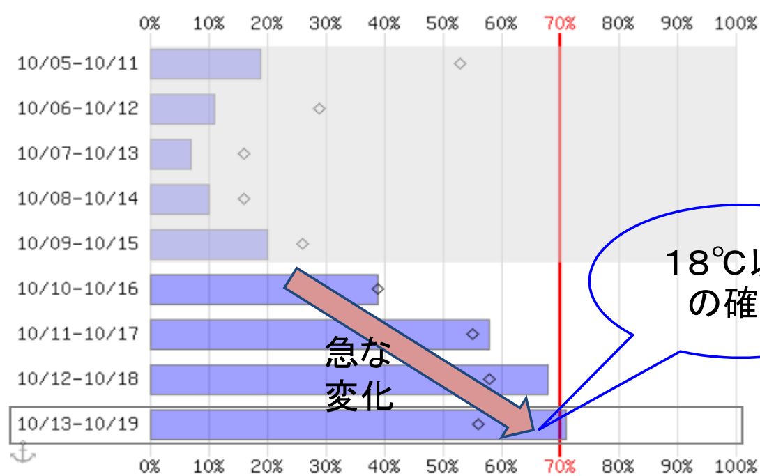
7日間平均気温の累積確率・確率密度分布図: 東京 (図の見方)
