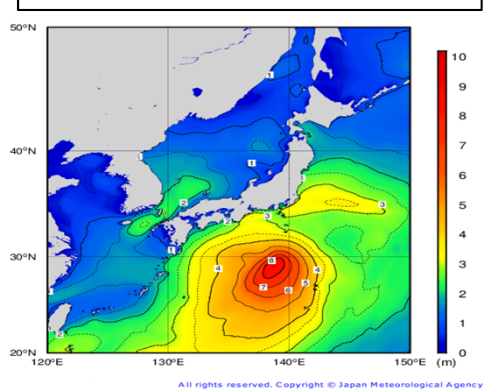
沿岸波浪 （実況図・予想図）
