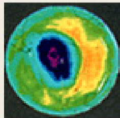
オゾンホール
