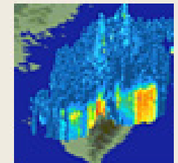
降雨立体構造
