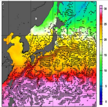
海水温・海流 (実況・予報)
