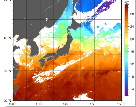
海面水温 (ひまわり9号の観測による)
