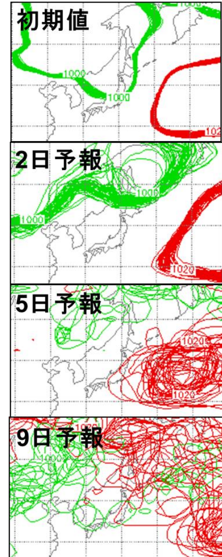
海面気圧の51個の 予報の重ね描き図
