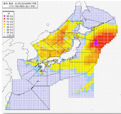
地方海上分布予報
